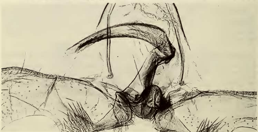
Figs 12-14. Male genitalia of Cydia Hb., aedeagus in situ. 12 - C. johanssoni sp.n., holotype, gen. prep. AB1991 ; 13 - C. blackmoreana (WALS.), gen. prep. R1991 ; 14 - C. blackmoreana (WALS.), gen. prep. S1991.
